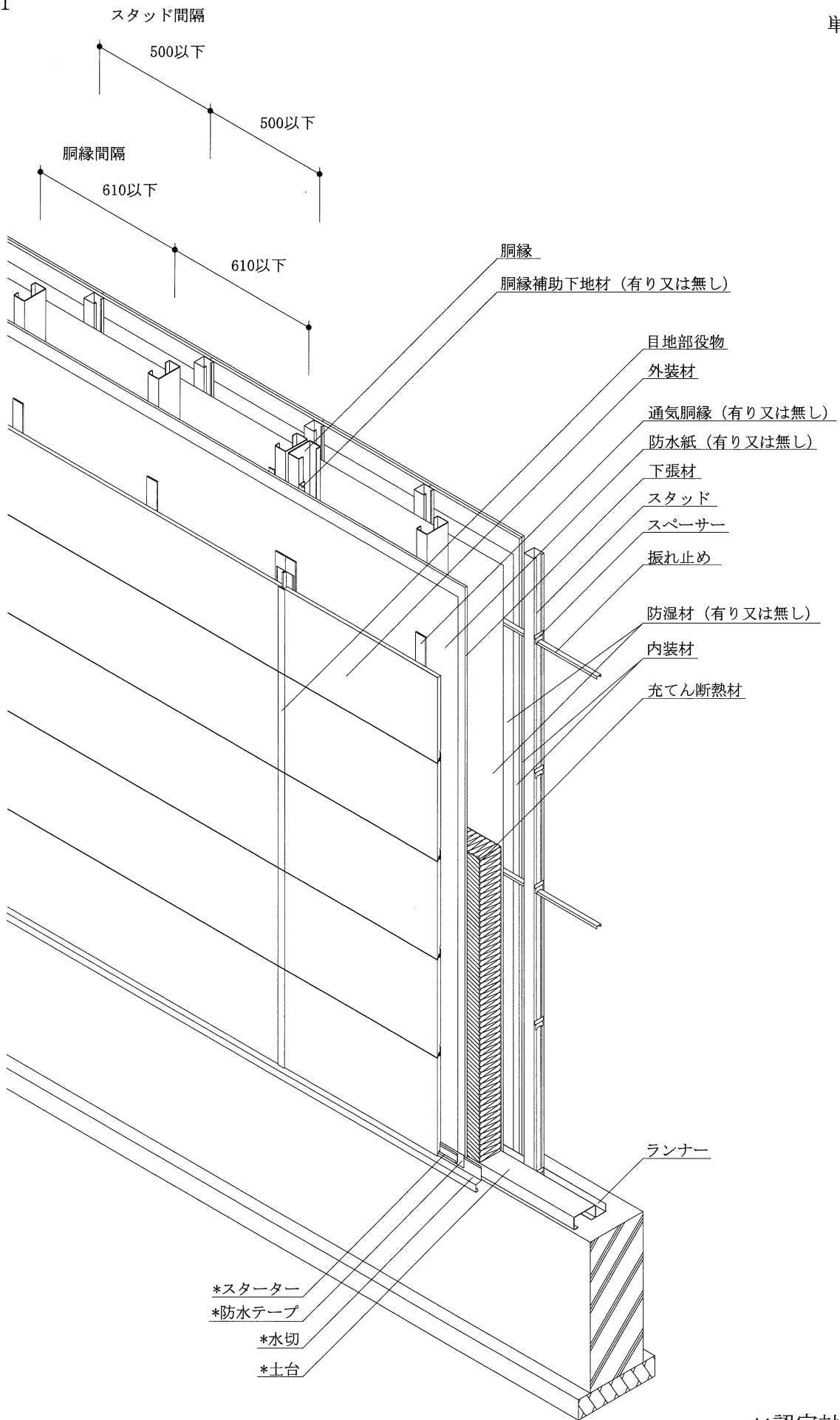
透視図 (別添-14)
