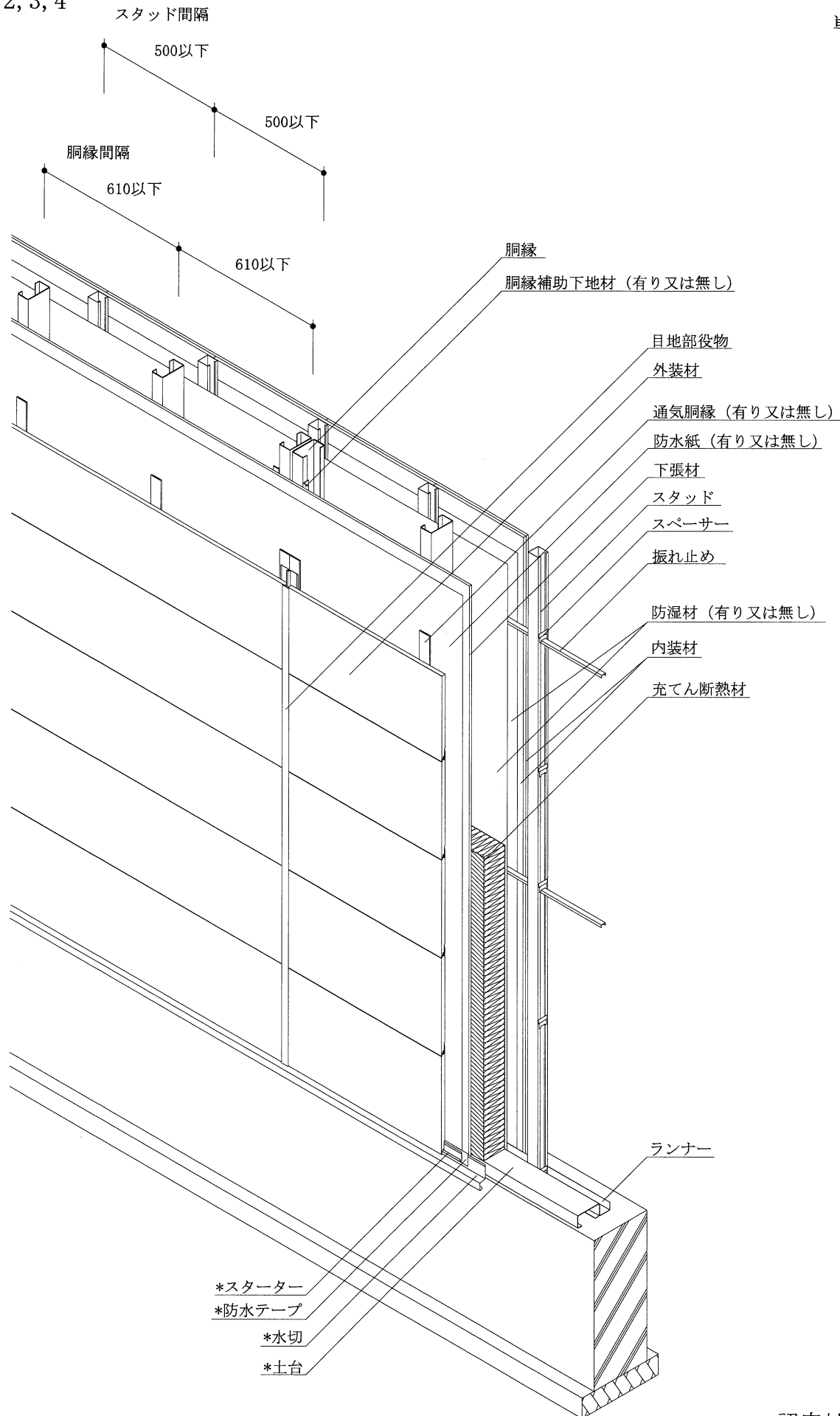
透視図 (別添-15)
